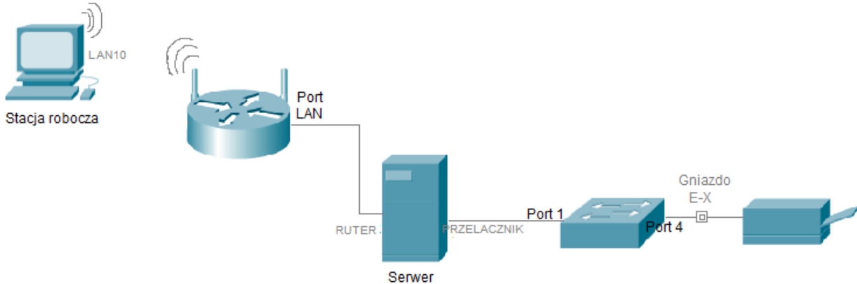
Schemat połączenia urządzeń
