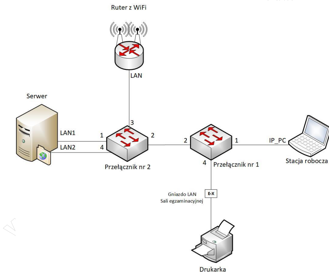
Schemat połączenia urządzeń
