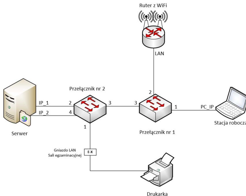
Schemat połączenia urządzeń
