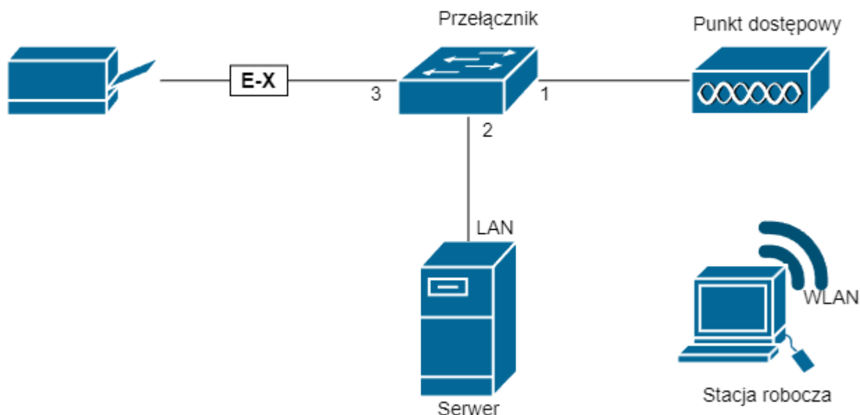
Schemat połączenia urządzeń
