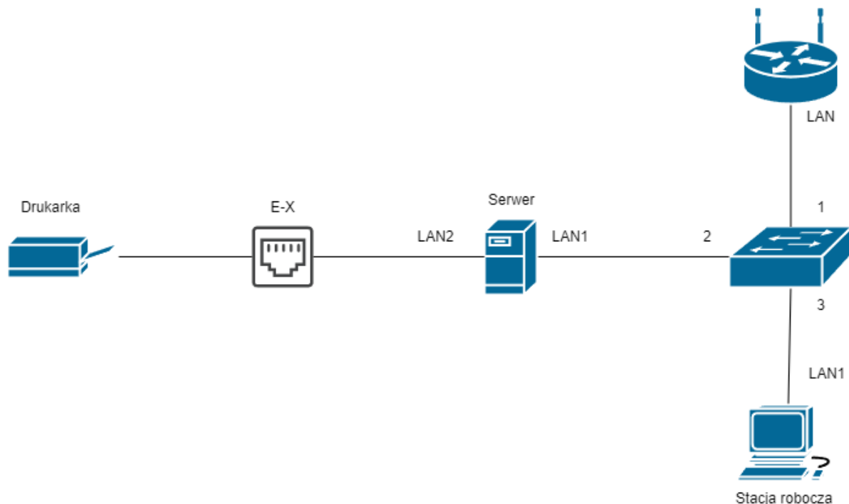
Schemat połączenia urządzeń
