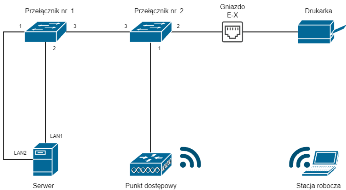
Schemat połączenia urządzeń
